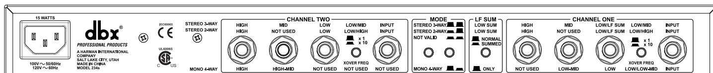
Face arrière du dbx 234s
