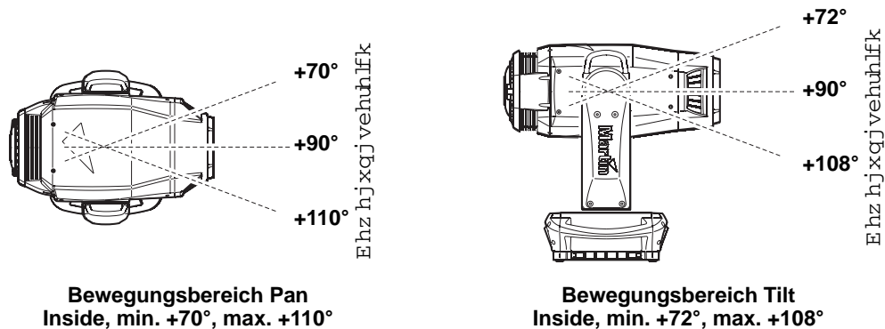
Bild 10: Pan/Tilt Begrenzung
