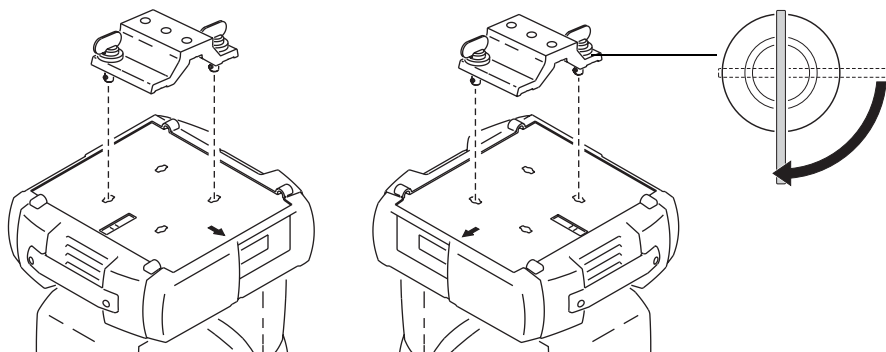
Bild 3: Klemmenadapter
