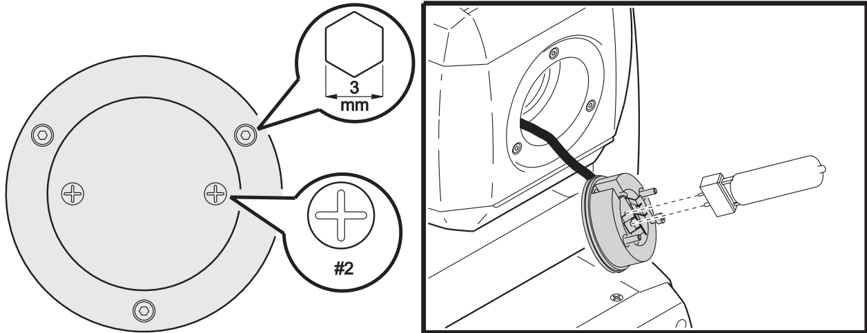
Bild 1: Installation des Leuchtmittels
