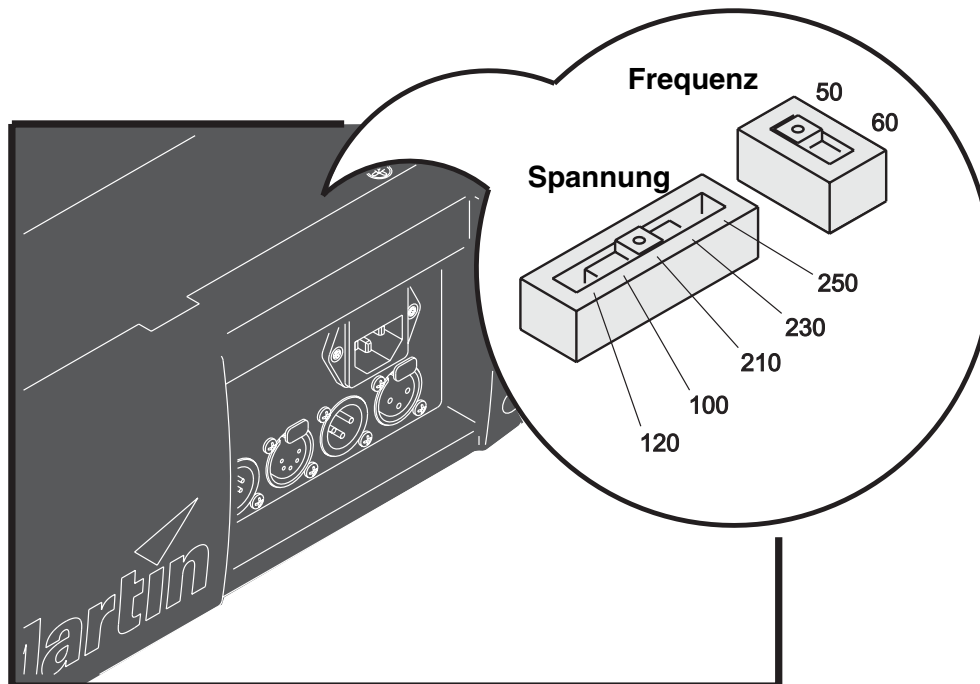
Bild 2: Einstellen des Netzteils
