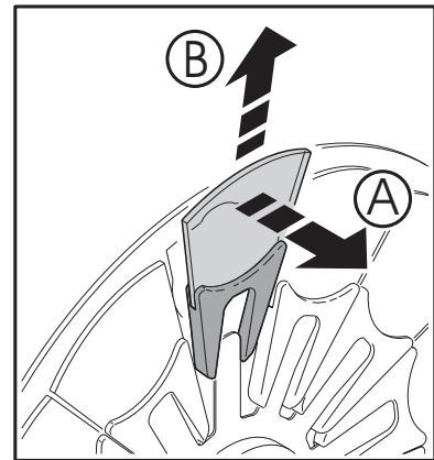
Bild 5: Austauschen eines Farbfilters
