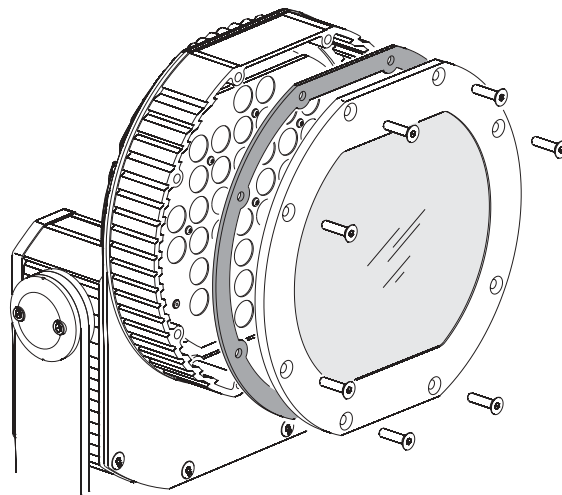
Bild 17: Schrauben und Dichtung der vorderen Abdeckung
