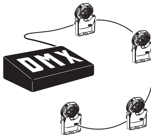
Bild 7: DMX Datenlinie
