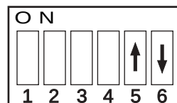
Normale Dipschalterstellung
