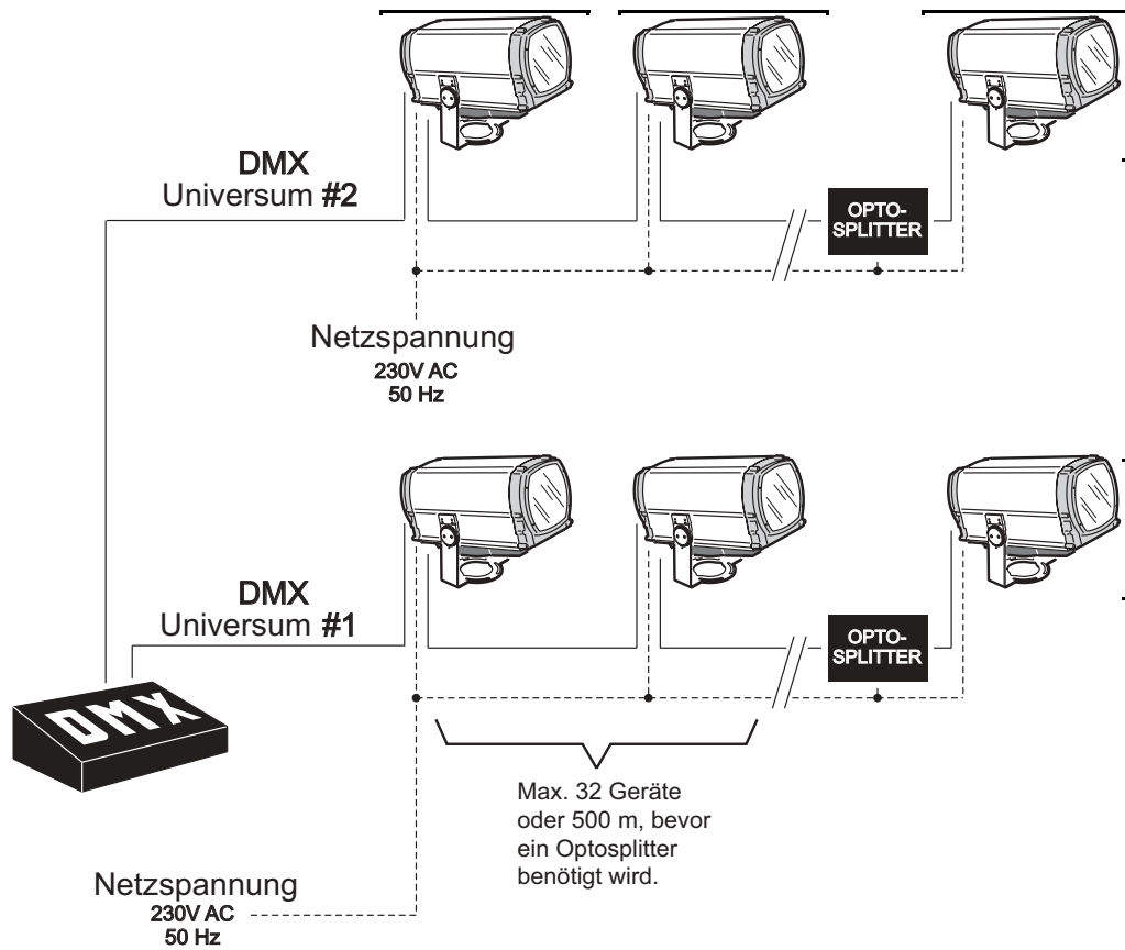
Bild 3: Verlegung der Netz- und Datenleitungen
