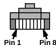
Bild 8: RJ-45 Pin-Identifizierung
