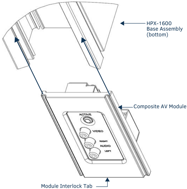
FIG. 6 INSERTING THE COMPOSITE AV MODULE INTO THE HPX-1600 CHASSIS
