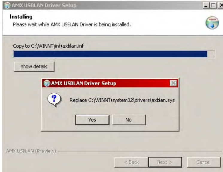
FIG. 7 Replace AXBLAN.SYS
