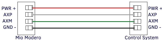
FIG. 4 AXLINK WIRING
