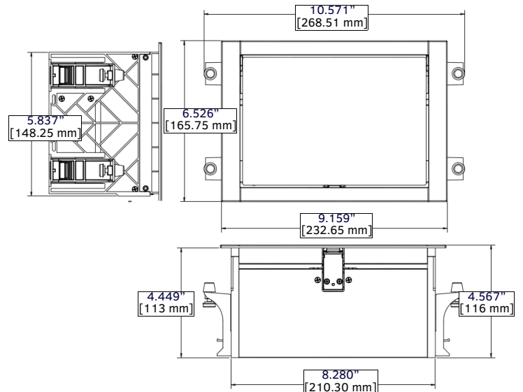
FIG. 3 HPX-MSP-7 DIMENSIONS
